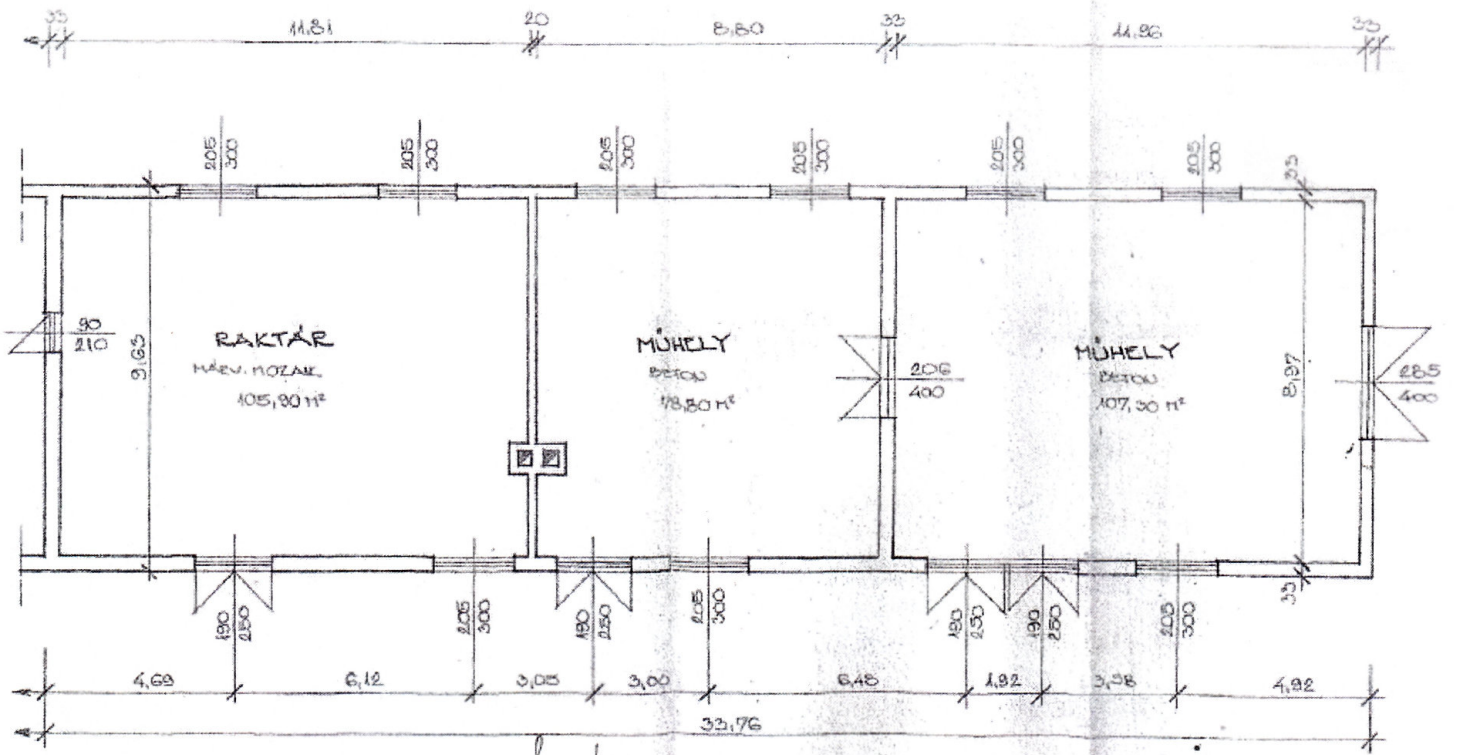
L. ÉPÍTŐ MŰHELY - ÉS RAKTÁR ALAPRAJZ M = 1/100
